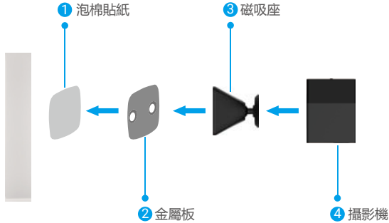
圖 1 使用泡棉貼紙安裝
