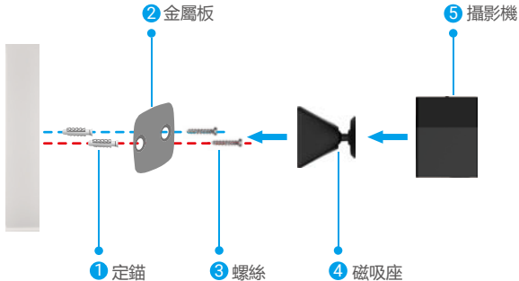
圖 2 使用螺絲安裝
